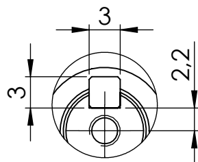
DETALHE D ESCALA 2 : 1
