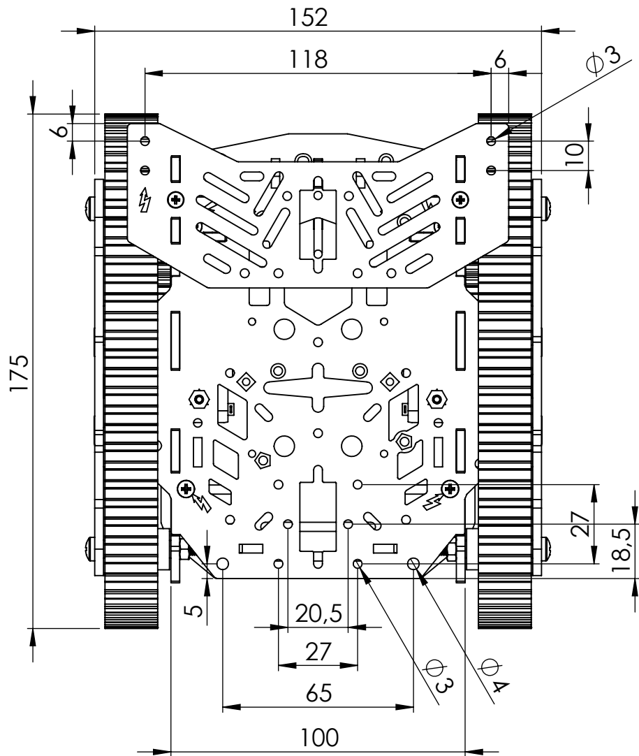
Dimensões & Fixações
