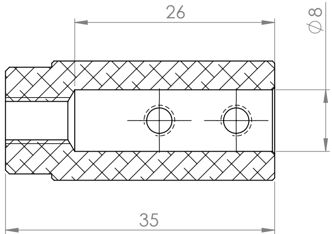
SEÇÃO B-B
