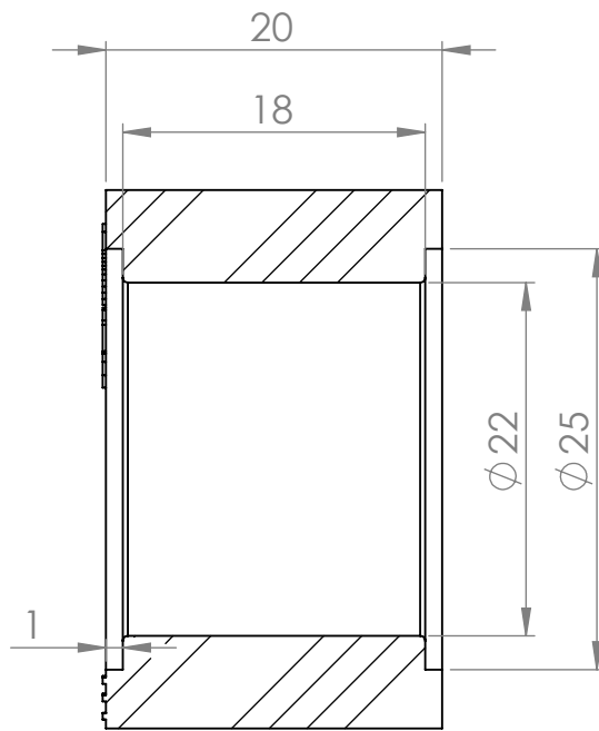
SEÇÃO G-G ESCALA 2 : 1
